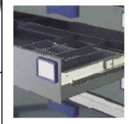
Accuride® Teleskopschienen in einem Transporter – Typ 3607. Teleskopschiene mit Verriegelung in geöffneter Position
